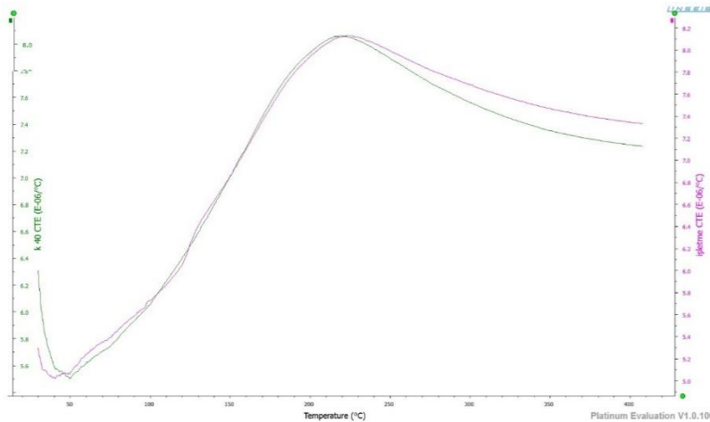
Şekil 3. K – 40 denemesi ve işletme çamurunun CTE genleşme grafikleri kıyaslaması
