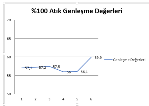
Şekil 3. %100 Atık denemeleri genleşme grafiği
