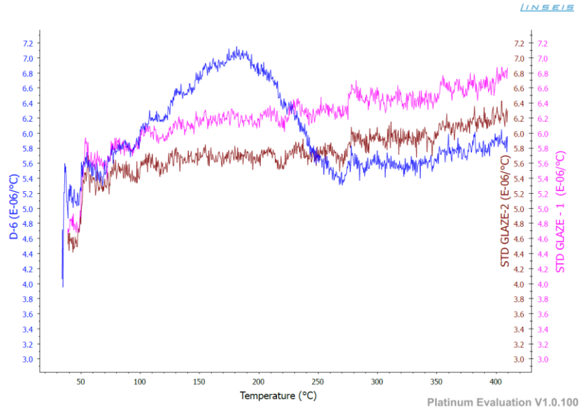
Şekil 2. D-6 reçetesi ile STD Glaze -1 ve STD Glaze-2 genleşme grafikleri - (D-6 59,9 \text{ e}^{-07}/\text{K} , STD Glaze – 1 61,8 \text{ e}^{-07}/\text{K} STD Glaze – 2 57,3 \text{ e}^{-07}/\text{K} )
