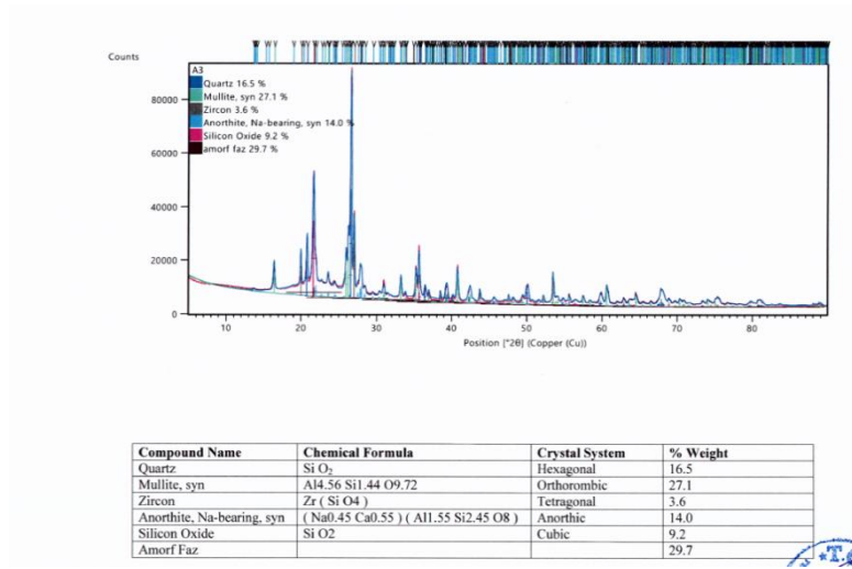
Şekil 8. %77 atık içeriğine sahip A-3 reçetesine ait X-Işını Kırınımı (XRD) analizi sonucu.
