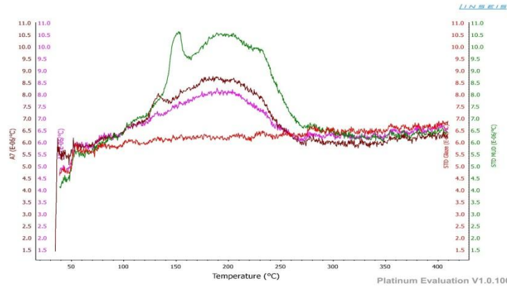
Şekil 11. A-3 reçetesi, A-7 reçetesi ve STD Mud, STD Glaze genleşme grafikleri (A-3 66,4 \times 10^{-7}/K , A-7 67,3 \times 10^{-7}/K , STD Glaze – 161,8 \times 10^{-7}/K , STD Mud – 274,8 \times 10^{-7}/K )
