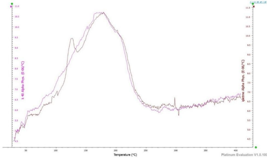
Şekil 2. K – 40 denemesi ve işletme çamurunun alfa fiziksel genleşme grafikleri kıyaslaması
