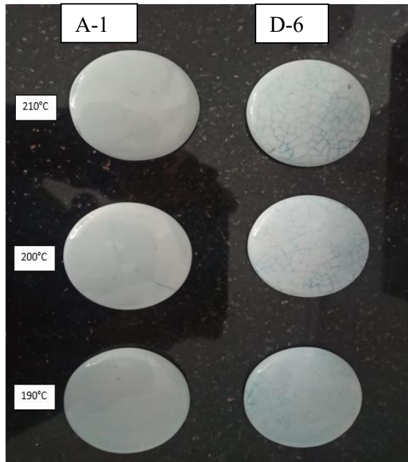
Şekil 5. A-1 ve D-6 reçetelerinden yapılan deneme kapaklarına uygulanan harkort testi.
