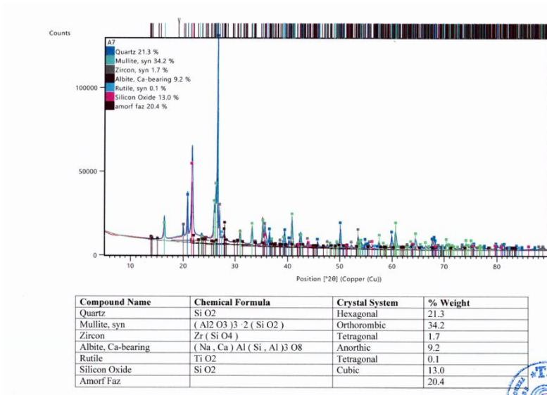
Şekil 9. %50 atık içeriğine sahip A-7 reçetesine ait X-Işını Kırınımı (XRD) analizi sonucu.
