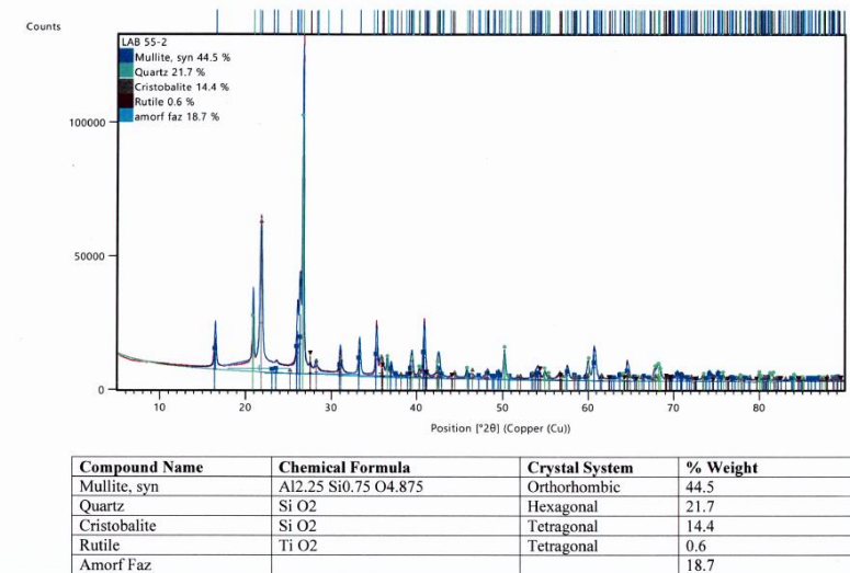
Şekil 10. STD 55-2 reçetesine ait X-Işını Kırınımı (XRD) analizi sonucu.
